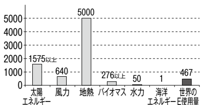
図2 現代技術による再生可能エネルギー資源の利用可能量と2009年の世界の年間エネルギー使用量(EJ/年)
