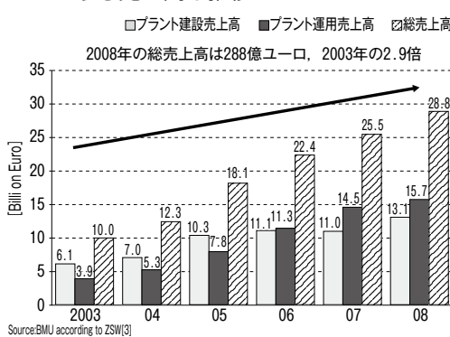
図3 ドイツの再生可能エネルギー産業における売上高の推移
