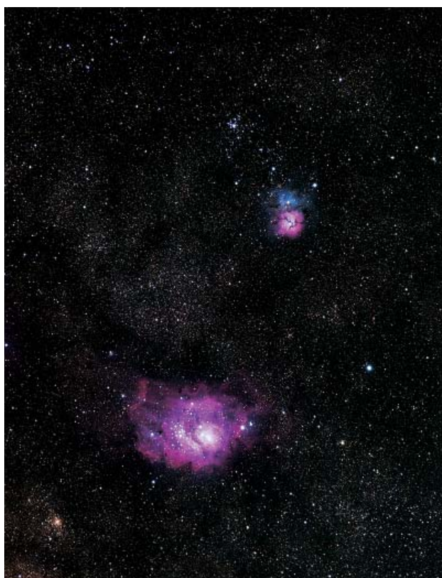
「千渦星雲と三裂星雲」
